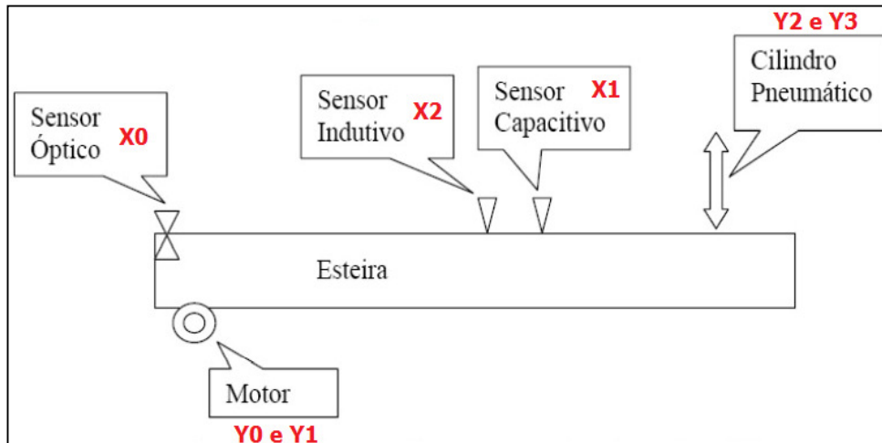
Figura 1. Esteira para a seleção de peças
